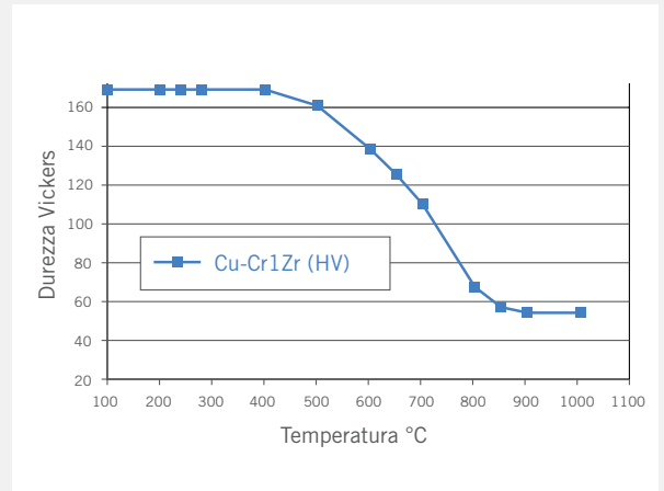
A-Trode ® – Variazione della durezza in funzione della temperatura
